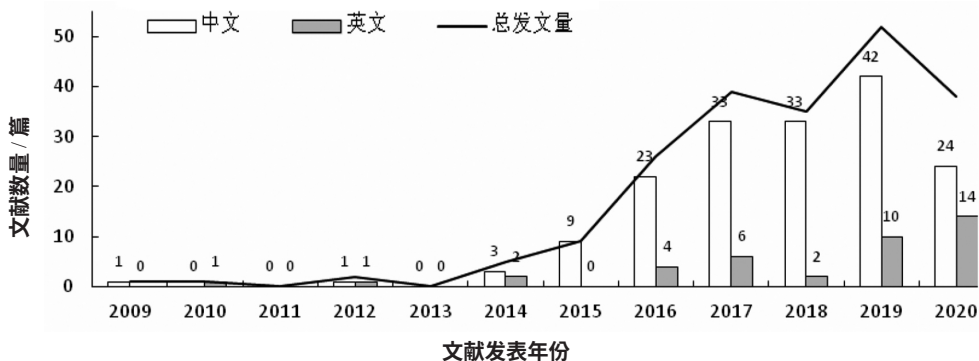
图 1 供应链集中度领域文献的时间分布
