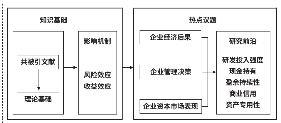
图3 供应链集中度整合研究框架
